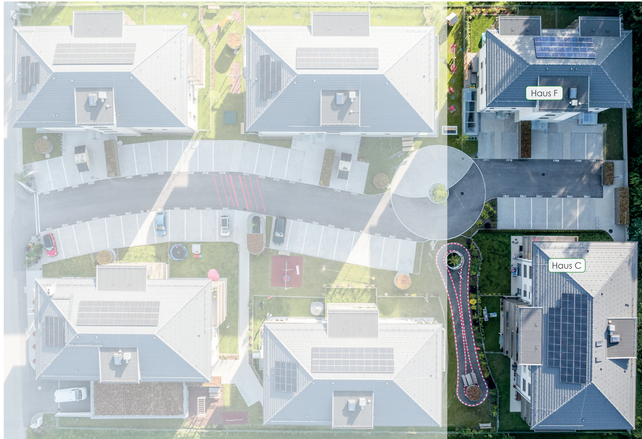
Haus C: HWB 28kWh/m 2 a; fGEE 0,62 | Haus F: HWB 32 kWh/m 2 a; fGEE 0,65
