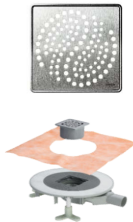
Bodenablauf Edelstahl Einlaufrost (oder gleichwertiges)
